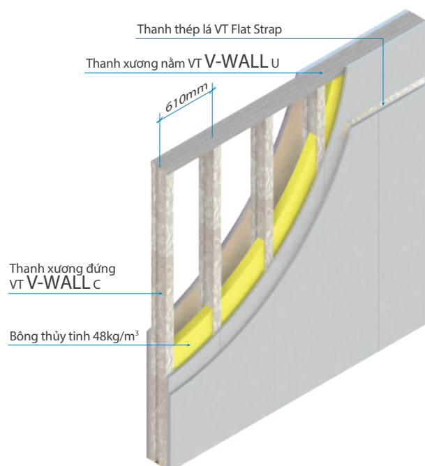
Tấm Thạch Cao VĨNH TƯỜNG-Gyproc Tiêu Chuẩn Áp dụng cho khu vực khô
